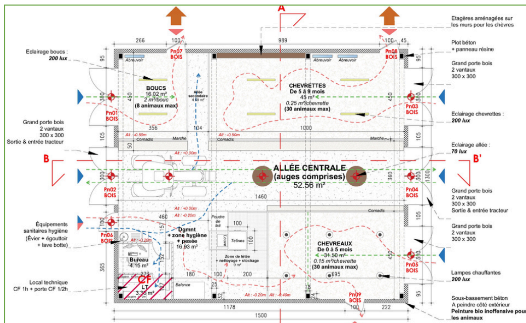
Plan du bâtiment chevette
